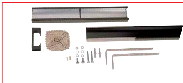
Extensie de sină 1600 mm pentru Kit-urile Marathon si Marathon Tiga cod 1615V000
